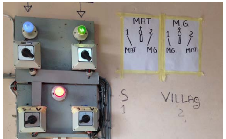
Système de «back up» et de bascule entre circuits d'alimentation
